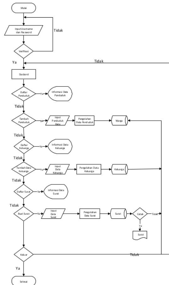
Gambar 2. Flowchart Sistem Baru
