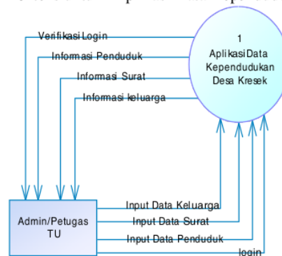
Gambar 3. Diagram Konteks
